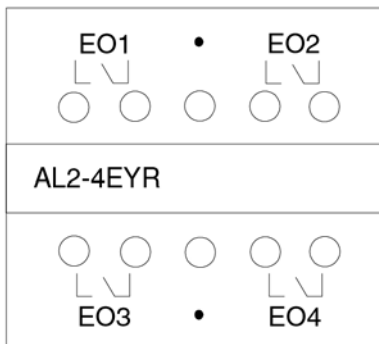
Рисунок 5.7: Устройство AL2-4EYR, выходные клеммы реле
