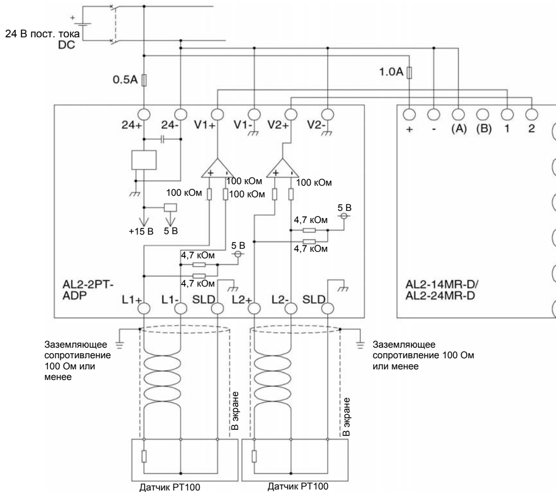
Рисунок 12.4: Электрические соединения
