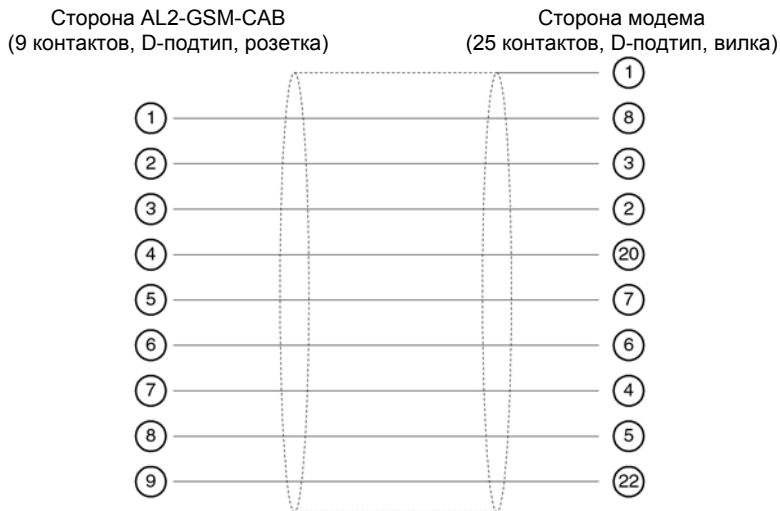
Рисунок 8.5: Схема прямого кабеля RS-232C между модемом и кабелем AL2-GSM-CAB, для справки.
