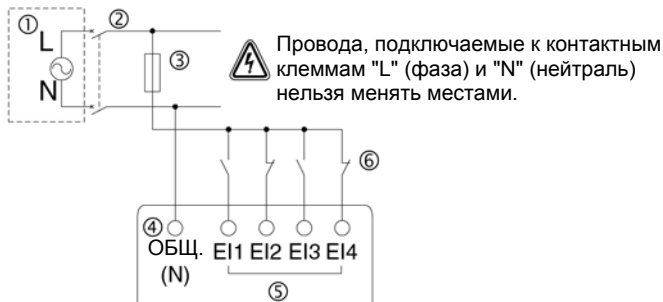
Рисунок 4.4: Схема электрических соединений с входными цепями, для AL2-4EX-A2
